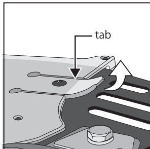
② 提起卡舌并拉出硬壳。 * 安装外壳时，提起卡舌并将外壳完全插入。
