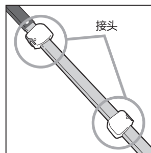
⑤ 有两个接头。操作步骤相同。
